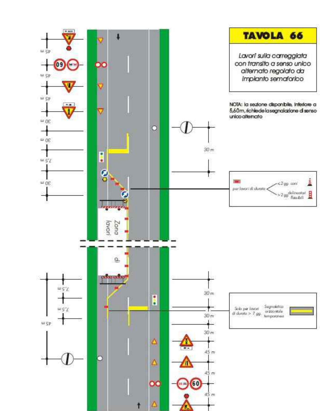
SCHEMA TIPO DELLA SEGNALETICA ( ESTRATTO D.M. 10/07/2002)
