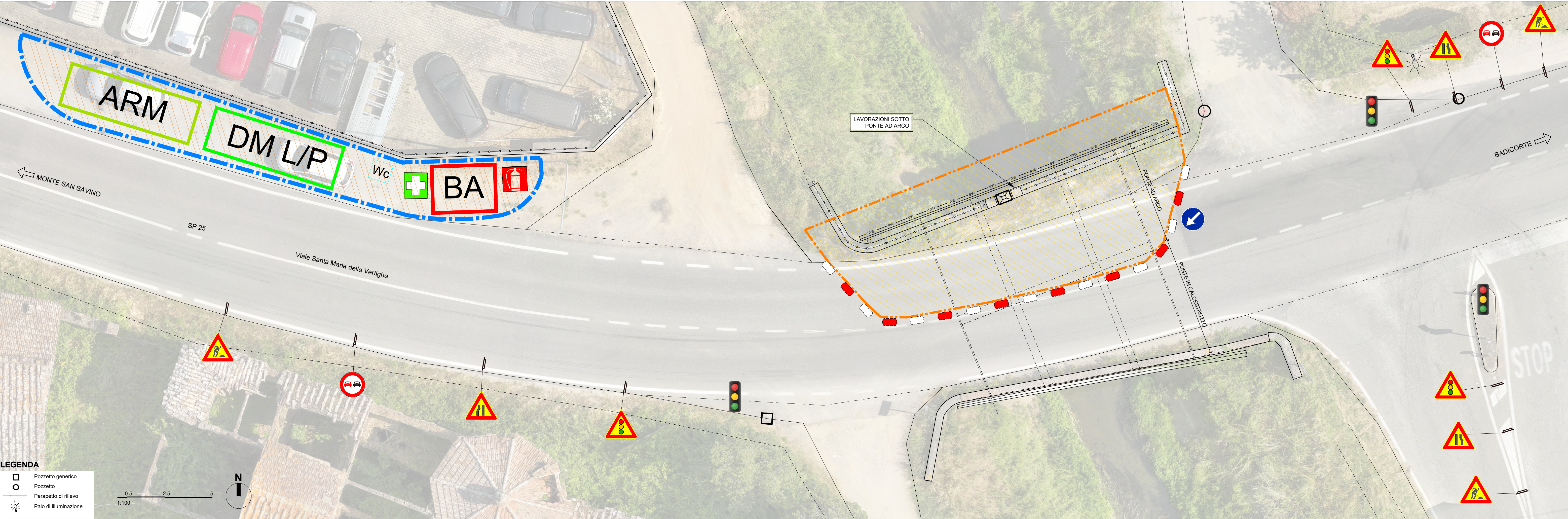
SCHEMA LAYOUT DI CANTIERE - FASE 2 | SCALA 1:100
