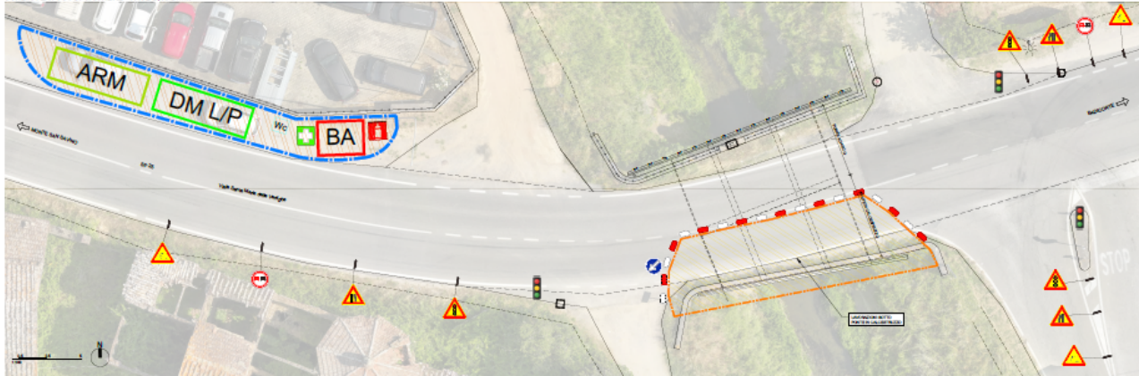
SCHEMA LAYOUT DI CANTIERE - FASE 2: SCALA 1:100
