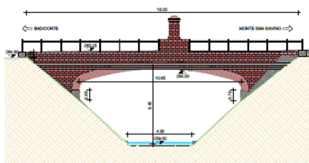
PROSPETTO PONTE AD ARCO LATO NORD
