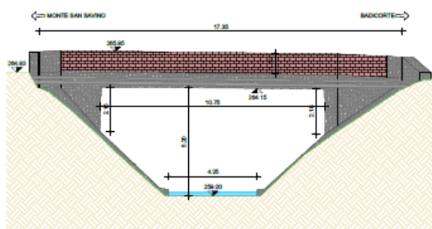
PROSPETTO PONTE IN CALCESTRUZZO LATO SUD
